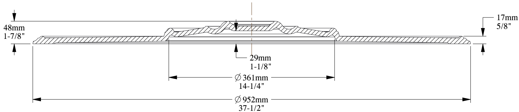
SECTION A-A SCALE 1:5
