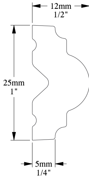
SCALE 2:1
